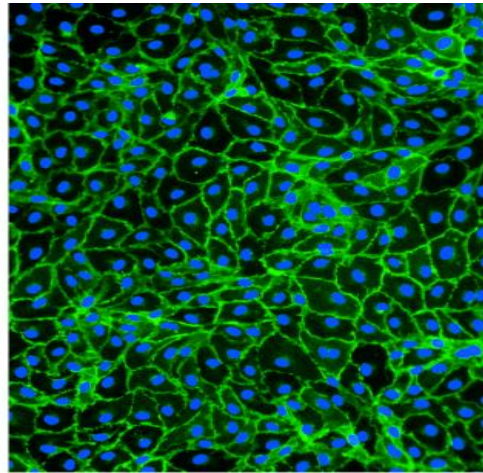
DAPI CD31
