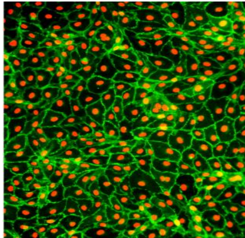
Prox1 CD31
